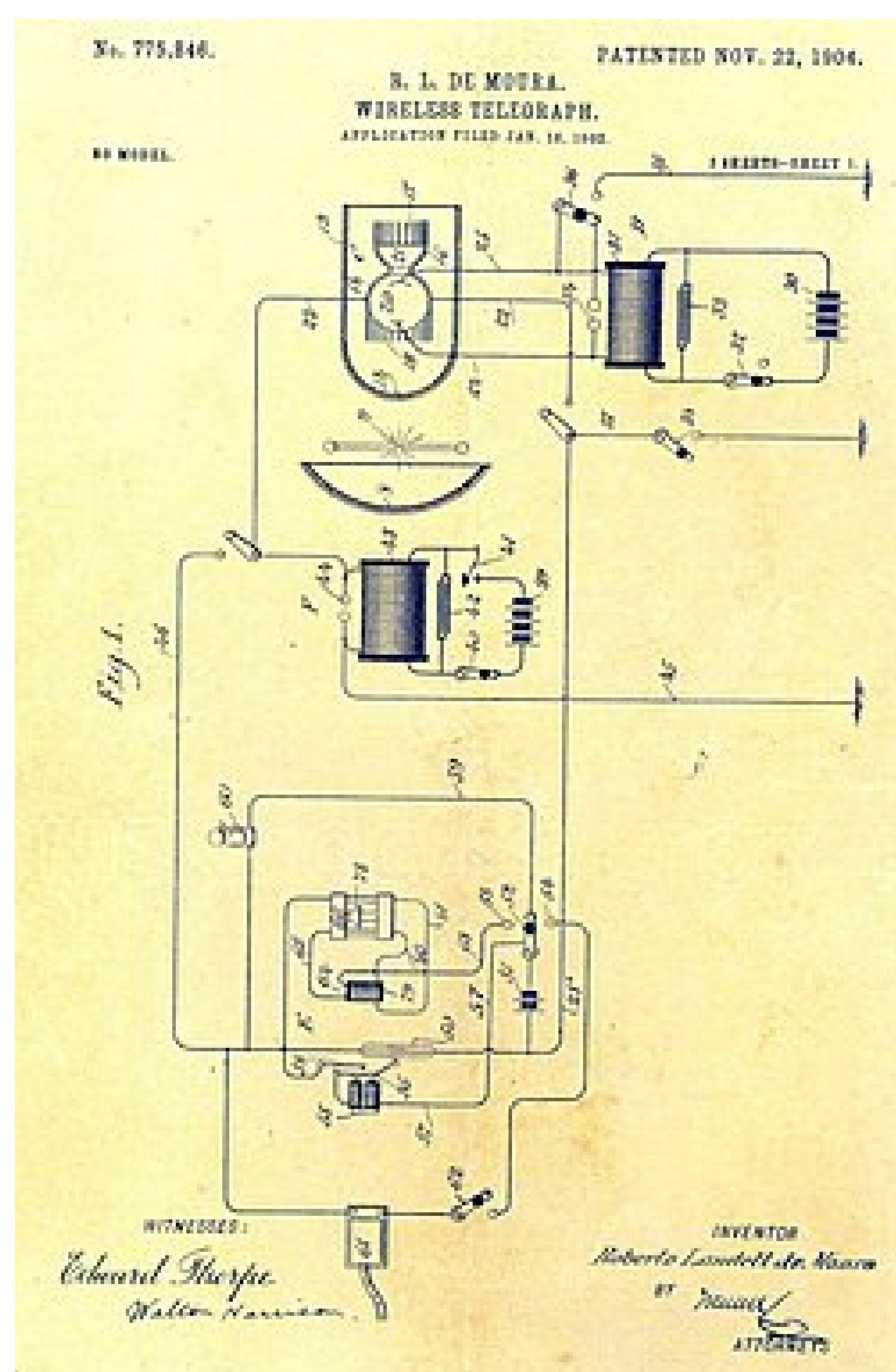
Esquema do telégrafo sem fio patenteado nos Estados Unidos em 1904 FONTE: https://pt.wikipedia.org/wiki/Roberto_Landell_de_Moura
