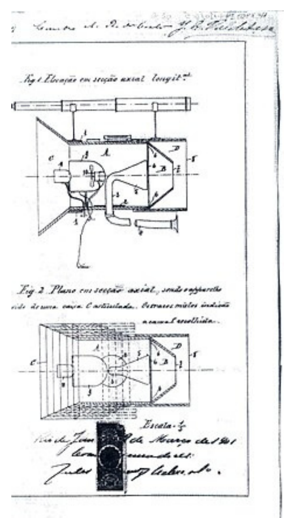
Esquema do telefone patentado no Brasil em 1901 FONTE: https://pt.wikipedia.org/wiki/Roberto_Landell_de_Moura
