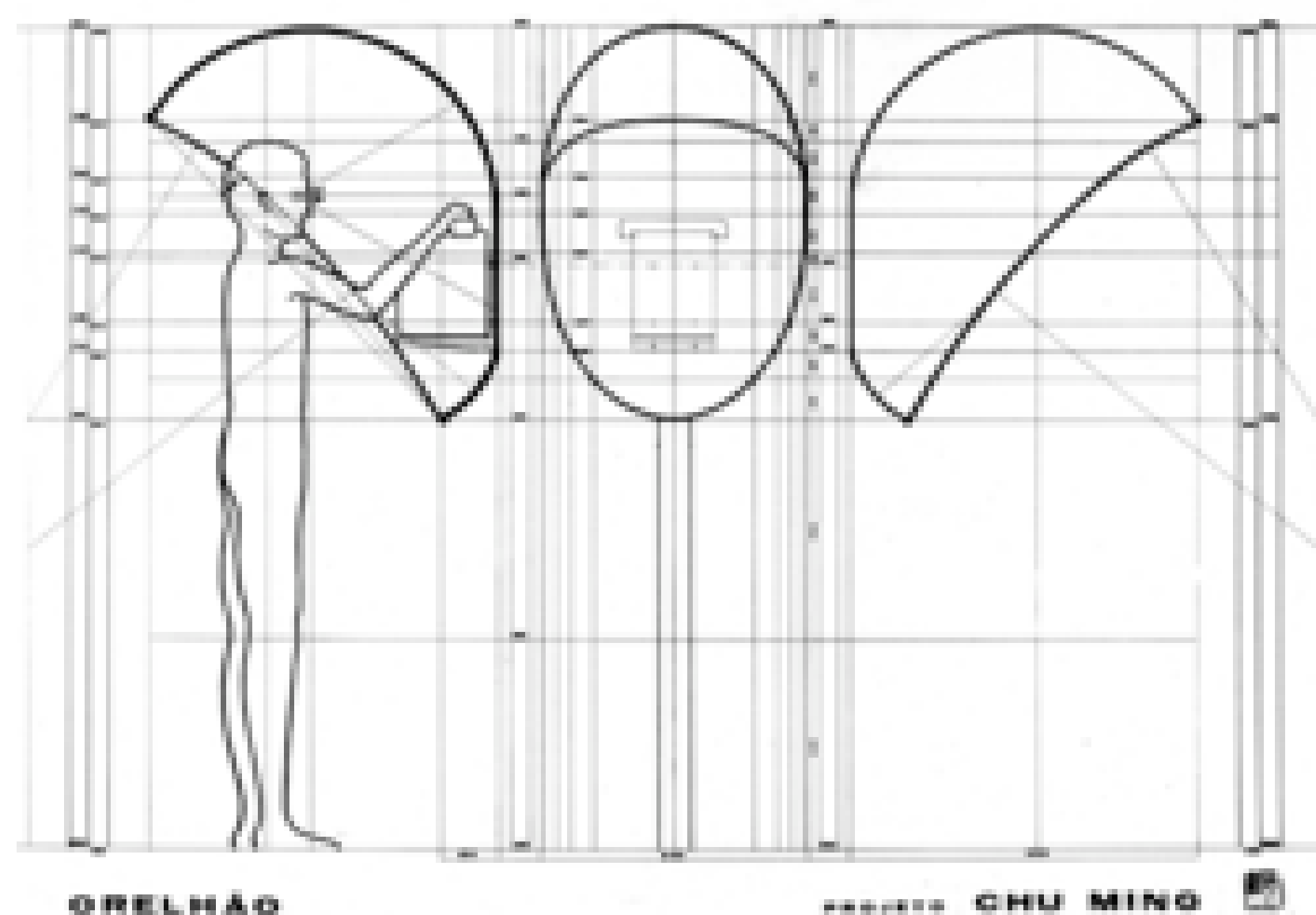
Projeto original do Orelhão FONTE: https://pt.wikipedia.org/wiki/Chu_Ming_Silveira
